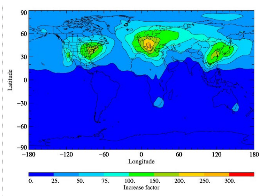
Abb. 1: Vorhergesagte TFA-Zunahme in der Troposphäre (die untersten 8 km der Atmosphäre) bei jährlichen R134a-Emissionen von 210.000 Tonnen pro Jahr und zukünftigen R1234yf-Emissionen in gleicher Höhe bei vollständigem Ersatz von R134a durch R1234yf [3]. Von Holland et al. werden für die Zukunft sogar noch höhere R1234yf-Emissionen prognostiziert (Nachdruck mit Genehmigung von ACS Earth & Space Chemistry. Copyright 2021 American Chemical Society.)
